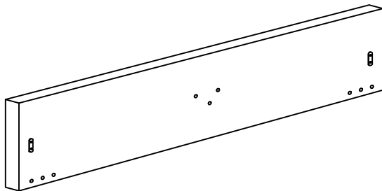
Footboard (P2)/Pied de pied (P2)
